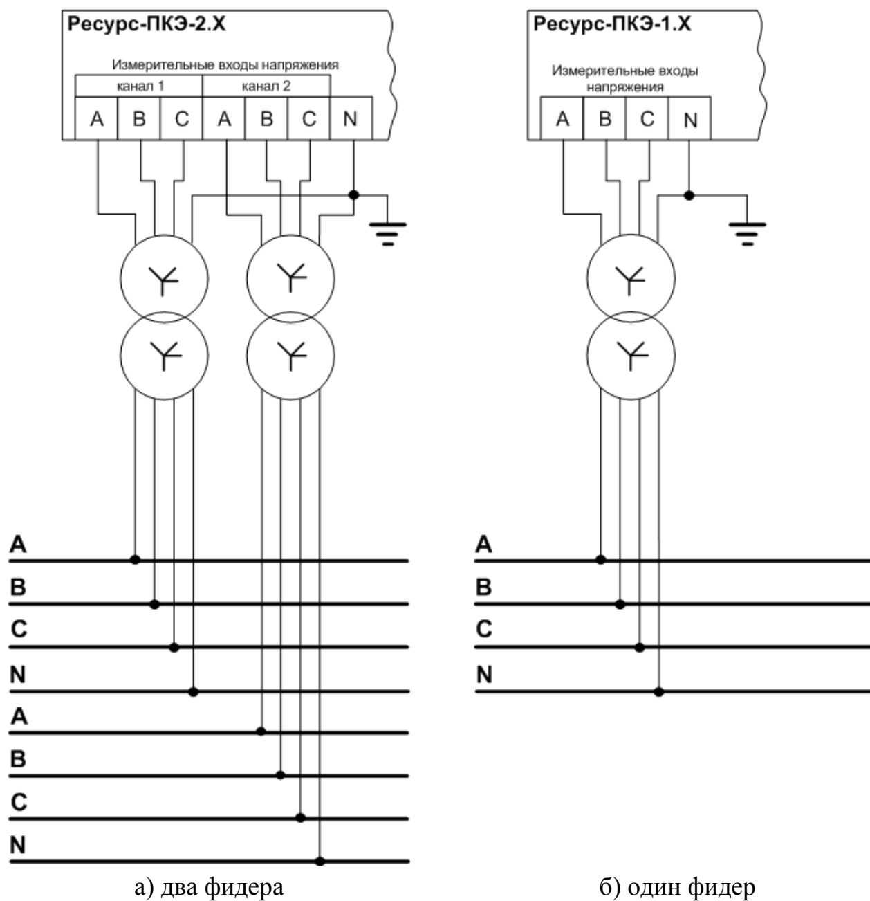
Рисунок В.5 - Трехфазная четырёхпроводная схема измерения напряжения с трехфазным измерительным трансформатором напряжения с выведенным нулем
