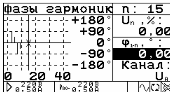
Рис. 4.13. Окно «Форма сигнала» в варианте представления «Фазы гармоник»
