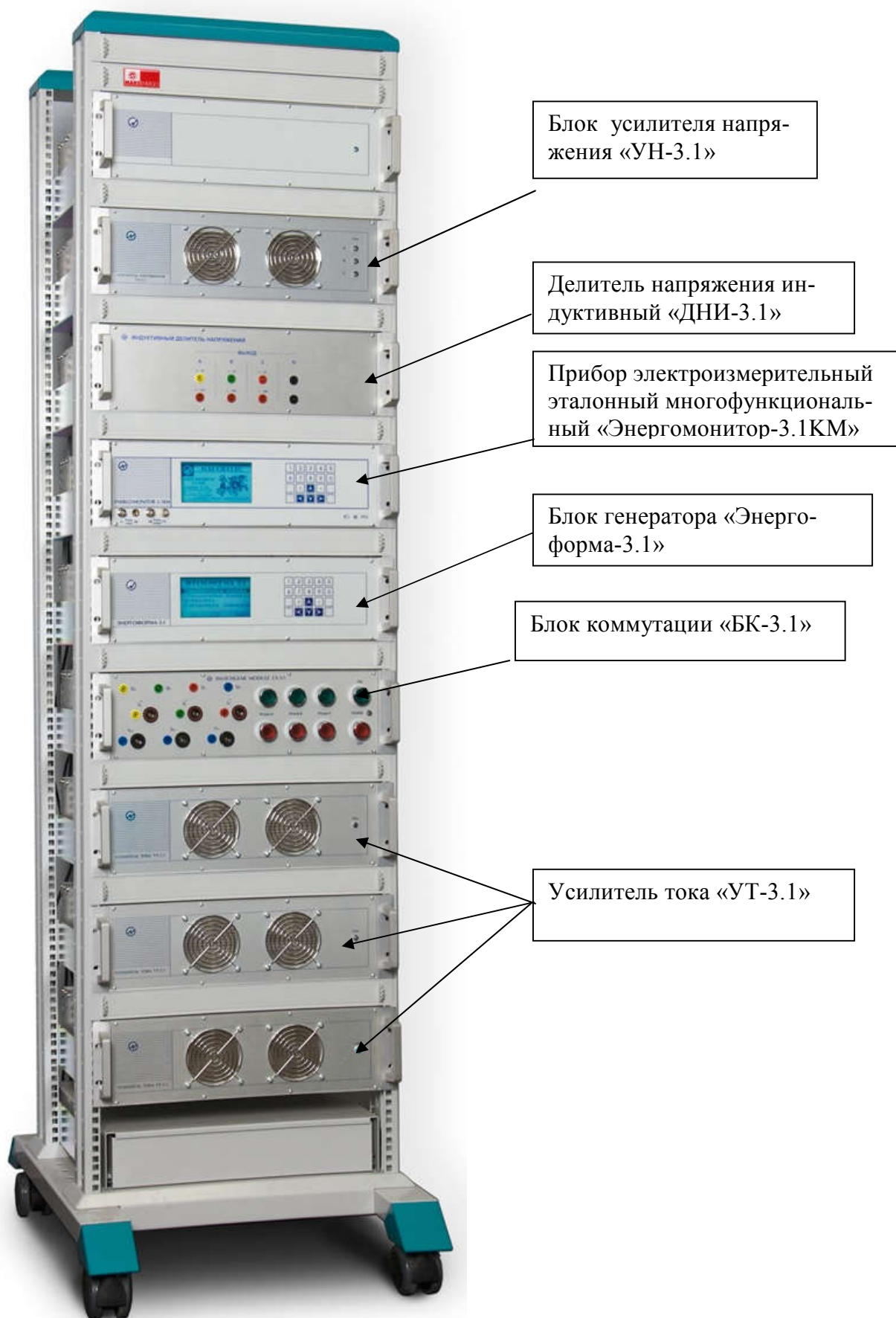
Рисунок 1. Установка "УППУ-МЭ 3.1КМ-С". Общий вид (Клеймо поверителя после поверки наносится на стационарную установку в виде наклейки на боковую стенку установки)
