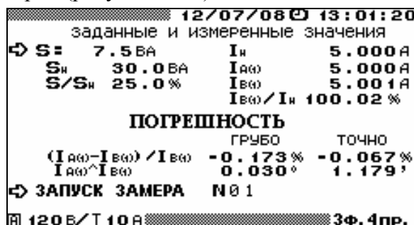
Рисунок 4.7.8 Окно результатов поверки ИТТ
