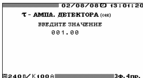
Рис. 4.8.13. Окно задания постоянной времени для режима «АМПЛИТУДНЫЙ ДЕТЕКТОР»
