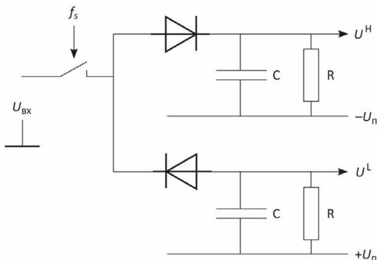
Рис. 4.53. Принцип обработки входного сигнала в режиме «АМПЛИТУДНЫЙ ДЕТЕКТОР»: U_{\text{ВХ}} — входное напряжение; f_s — частота дискретизации (12,8 кГц); U^H — значения огибающей напряжения сверху; U^L — значения огибающей напряжения снизу; \tau = RC — постоянная времени (задается в диапазоне от 0,1 до 100 с); -U_{\text{П}} — минимально возможное напряжение; +U_{\text{П}} — максимально возможное напряжение
