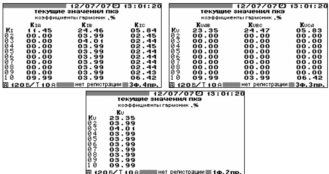
Рис. 4.24. Окна отображения коэффициентов искажения синусоидальности и гармонических составляющих напряжений и токов для различных схем включения
