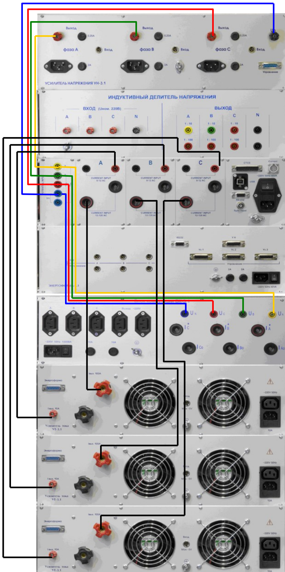
Рисунок А.5. Схема подключения Прибора «Энергомонитор-3.1КМ» к Установке
