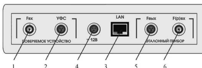
Рисунок 2.14 Передняя панель Преобразователя «ПТНЧ»
