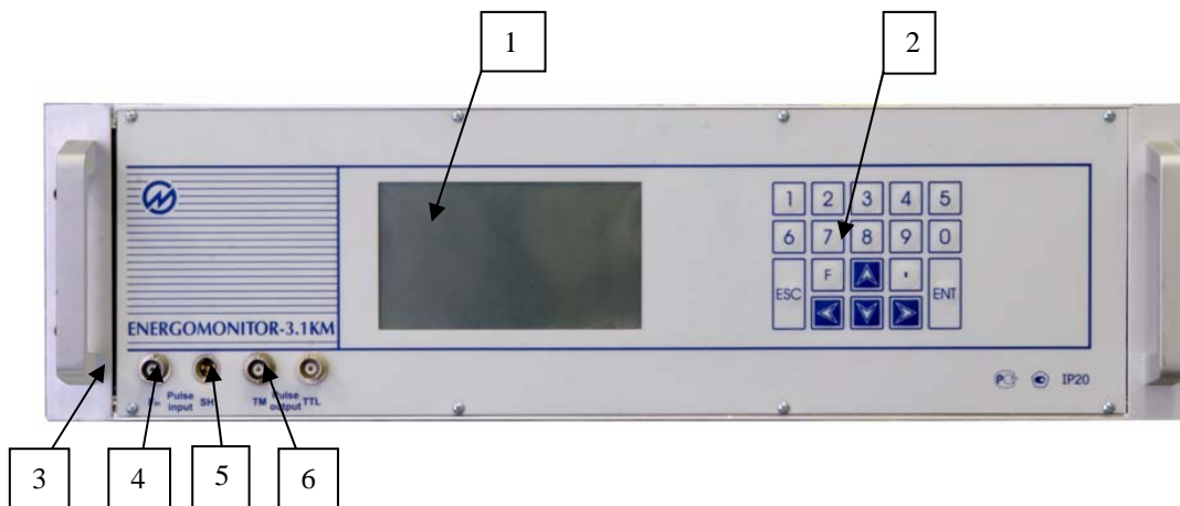
Рисунок 2.7 Вид лицевой панели прибора «Энергомонитор-3.1КМ»
