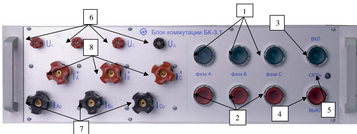
Рисунок 2.1 Вид лицевой панели блока коммутации «БК-3.1»
