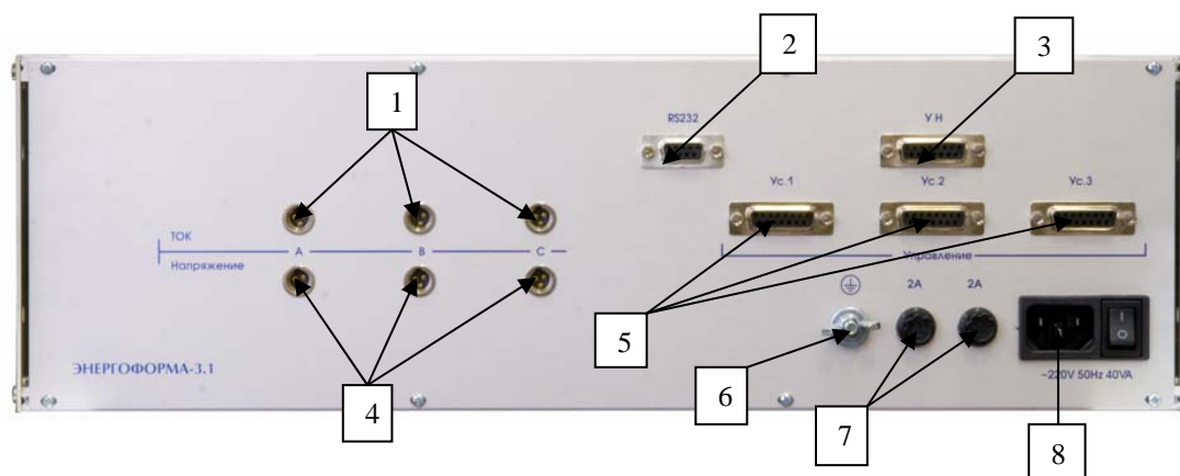
Рисунок 2.6 Вид задней панели блока генератора «Энергоформа-3.1» 1 — соединители для передачи форм сигналов тока на усилители; 2 — соединитель интерфейса RS-232; 3 — соединитель шины управления усилителями напряжения; 4 — соединители для передачи форм сигналов напряжения на усилители; 5 — соединители шин управления усилителями тока; 6 — соединитель заземления; 7 — держатели предохранителей; 8 — соединитель и тумблер питания
